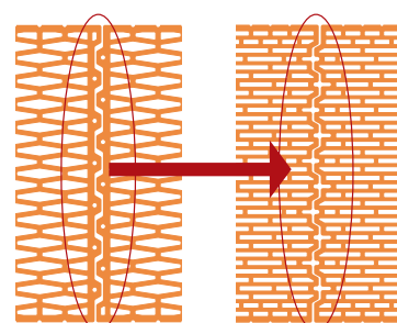
tradiční řešení spoje cihel Porotherm 44
