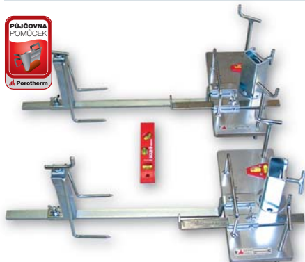
Vyrovňovací souprava pro založení první vrstvy broušených cihel
