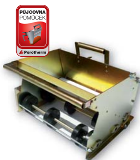
Maltovací vozík pro nanášení tenkovrstvé malty Porotherm Profi celoplošným způsobem
