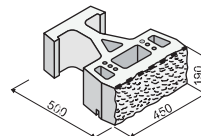
GEOSTONE® - FLAT štípaný rustik
