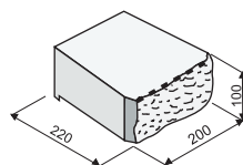
GARDEN STONE ŠTÍPANÝ RUSTIK
