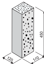
KB palisáda G-B 140-450
