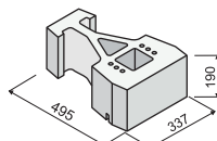
GEOSTONE® - FLAT třičtvrták hladký
