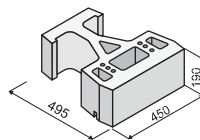
GEOSTONE® - FLAT hladký
