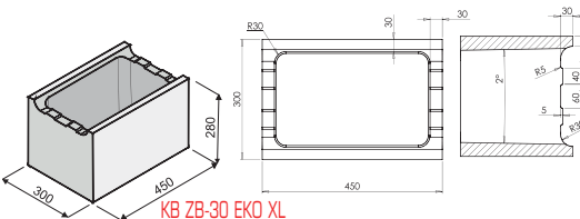
KB ZB-30 EKO XL
