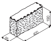
KB 9-11 B GRIND
