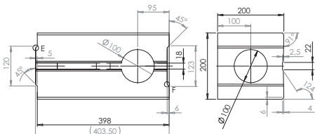
D-RainBlok rozdělovací "T"
