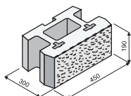
Pohledový prvek - CH štípaný
