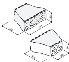
ZIQZAQ BLOK štípaný grind
