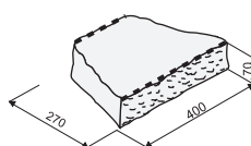
Nášlapný kámen poloviční
