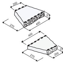
ZIQAQ BLOK 70 štípaný grind
