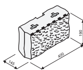
Pohledový prvek 400 štípaný grind
