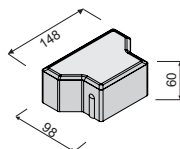
UNIKOST PŮLKA 60 mm
