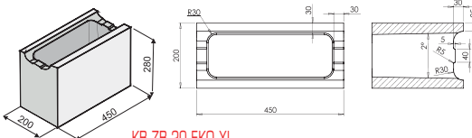
KB ZB-20 EKO XL
