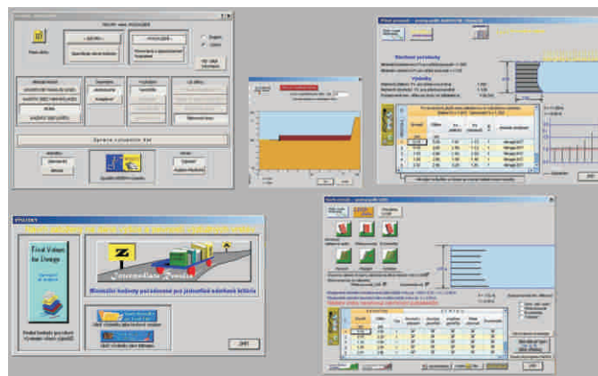
Výsledek návrhu vyztuže stěny
