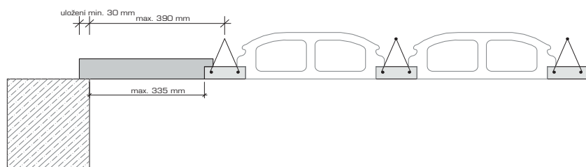
Řez stropem - stropní deska
