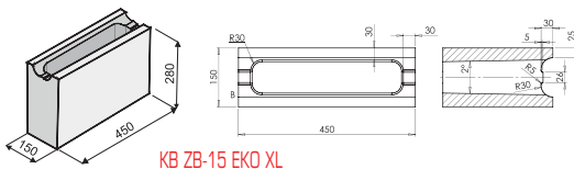
KB ZB-15 EKO XL
