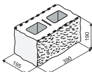
KB 7-21 B GRIND
