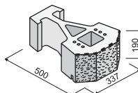
GEOSTONE® - BENT třičtvrták štípaný
