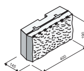
Pohledový prvek 400 štípaný rustik
