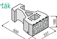
GEOSTONE® - FLAT třičtvrták štípaný
