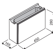
Lidovka hladká průběžná
