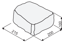
GARDEN STONE HLADKÝ GRIND
