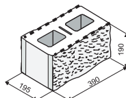
KB 7-21 B RUSTIK
