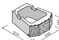
GEOSTONE® - SHELF štípaný
