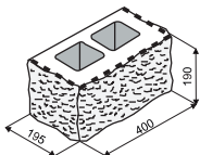
KB 9-21 B RUSTIK
