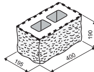
KB 13-21 B 400 RUSTIK
