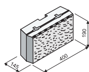
Pohledový prvek 400 štípaný
