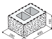
KB 15-21 B GRIND
