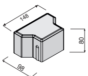
UNIKOST PŮLKA 80 mm
