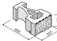
GEOSTONE® - FLAT třičtvrták štípaný rustik
