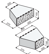
ZIQZAQ BLOK štípaný
