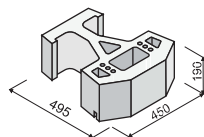
GEOSTONE® - BENT hladký
