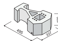
GEOSTONE® - BENT třičtvrták hladký
