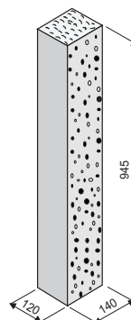
KB palisáda G-B 140-950
