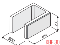
KBF 30 - 7 A-U
