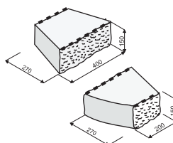
ZIQZAQ BLOK štípaný rustik
