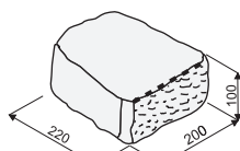
GARDEN STONE ŠTÍPANÝ GRIND
