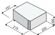
GARDEN STONE HLADKÝ
