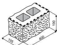
KB 9-21 B GRIND
