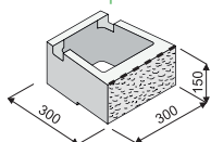
CUP STONE MALÝ – provedení štípané
