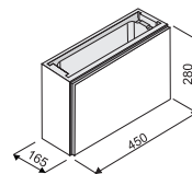
Lidovka hladká koncová
